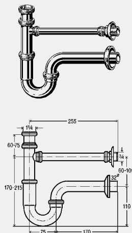
Cijevni sifon - kromirani mesing Oprema Prilagodljiva navojna spojnica, priključak za prodimu vodu, podesiva cijev 160 mm, odvodni luk 170 mm s nadzorom kvalitete prema DIN EN 274 Model 5611.02
