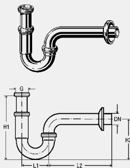
Cijevni sifon - kromirani mesing s nadzorom kvalitete prema DIN EN 274 Model 5611
