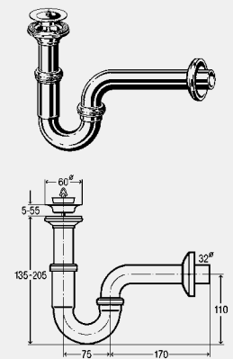
Cijevni sifon - kromirani mesing Oprema Univerzalni ventil od plemenitog čelika, čep ventila, brtva za gornji dio ventila, prilagodljiva cijev 100 mm, odvodni luk 170 mm s nadzorom kvalitete prema DIN EN 274 Model 5612
