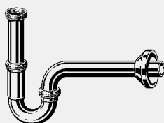
Cijevni sifon Plus-sifon - mesing Oprema Prilagodljiva cijev 120 mm, odvodni luk 220 mm s nadzorom kvalitete prema DIN EN 274 Model 5611.5
