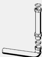
Odvodno koljeno 90° - umjetni materijal Oprema Ispusna cijev Model 5632.2
